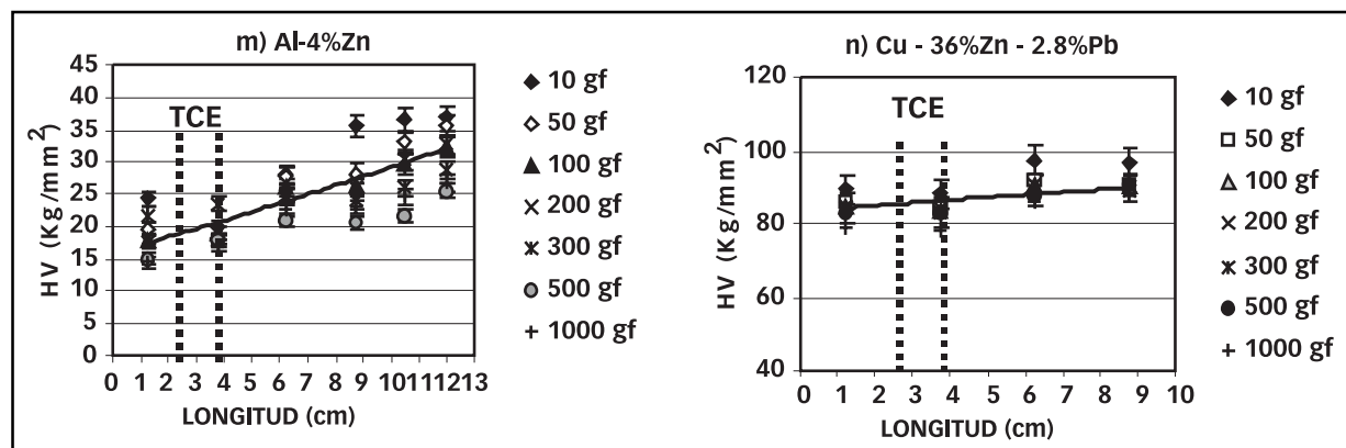
FIGURA 2: Valores de microdureza en función de la longitud de las probetas empleando diferentes cargas. a-e) Al-Cu. f-h) Al-Si. i) Al-Li. j-k) Al-Mg. l-m) Al-Zn. n) Cu-Zn.
