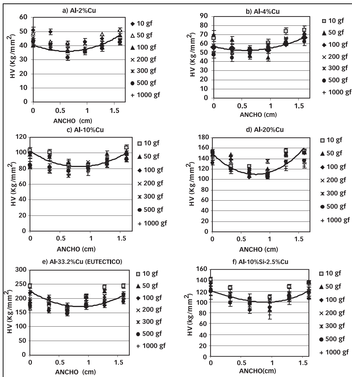
FIGURA 2: Valores de microdureza en función de la longitud de las probetas empleando diferentes cargas. a-e) Al-Cu. f-h) Al-Si. i) Al-Li. j-k) Al-Mg. l-m) Al-Zn. n) Cu-Zn.
