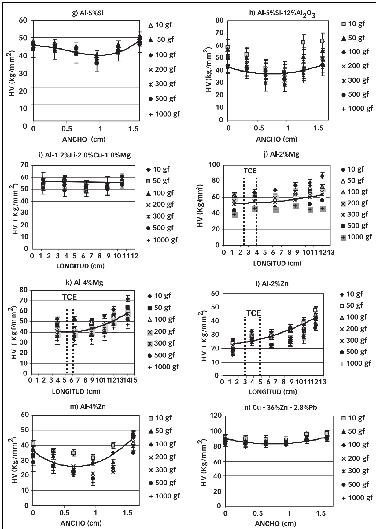
FIGURA 3: Valores de microdureza en función del ancho de las probetas empleando diferentes cargas. a-e) Al-Cu. f-h) Al-Si. i) Al-Li. j-k) Al-Mg. l-n) Al-Zn. n) Cu-Zn.
