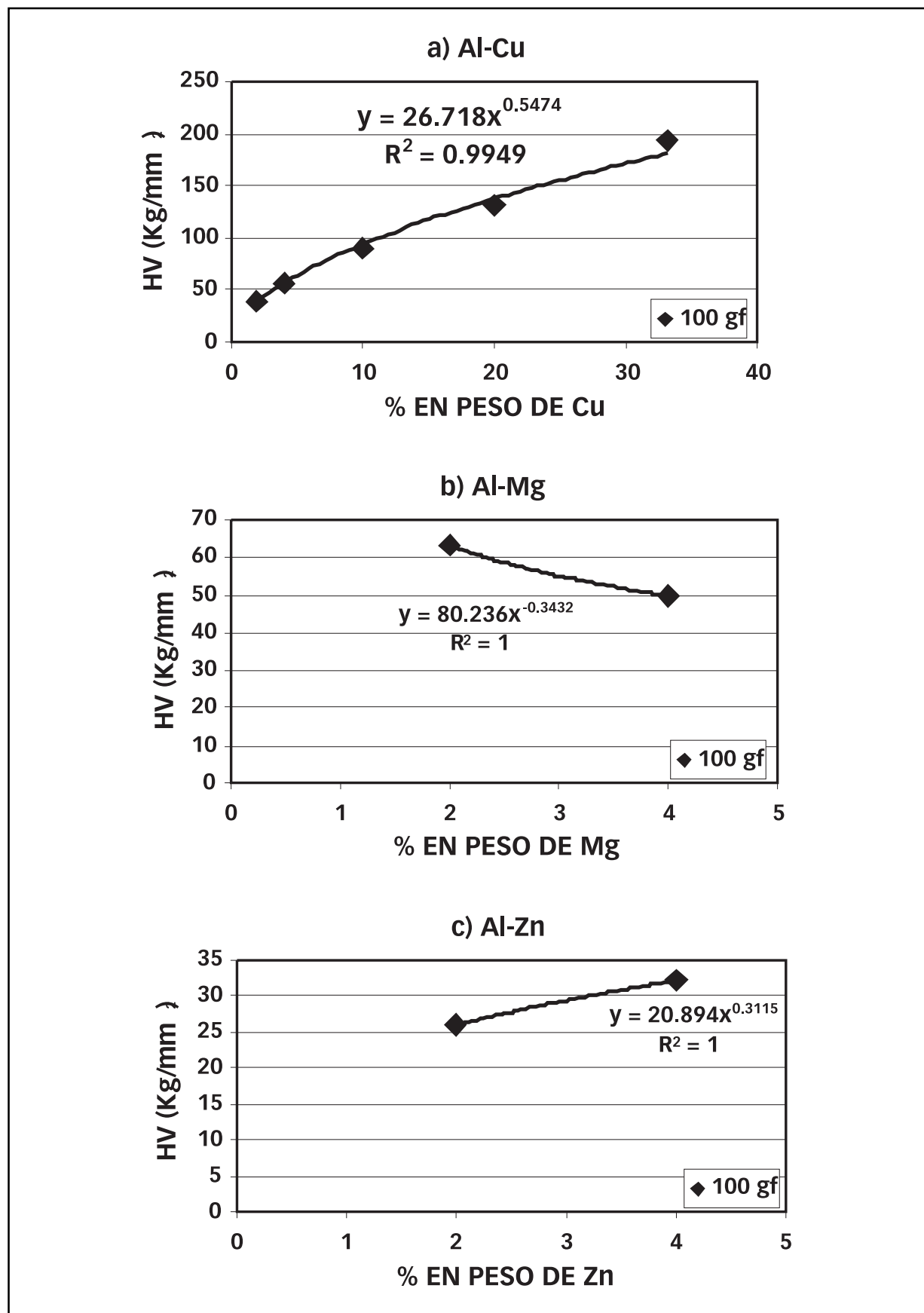
FIGURA 4: Valores de microdureza en función de la concentración utilizando una carga de 100 gf. a) Al-Cu. b) Al-Mg. c) Al-Zn.
