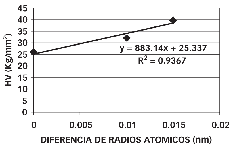
FIGURA 6: Valores de microdureza en función de la diferencia de radios atómicos utilizando una carga de 100 g.
