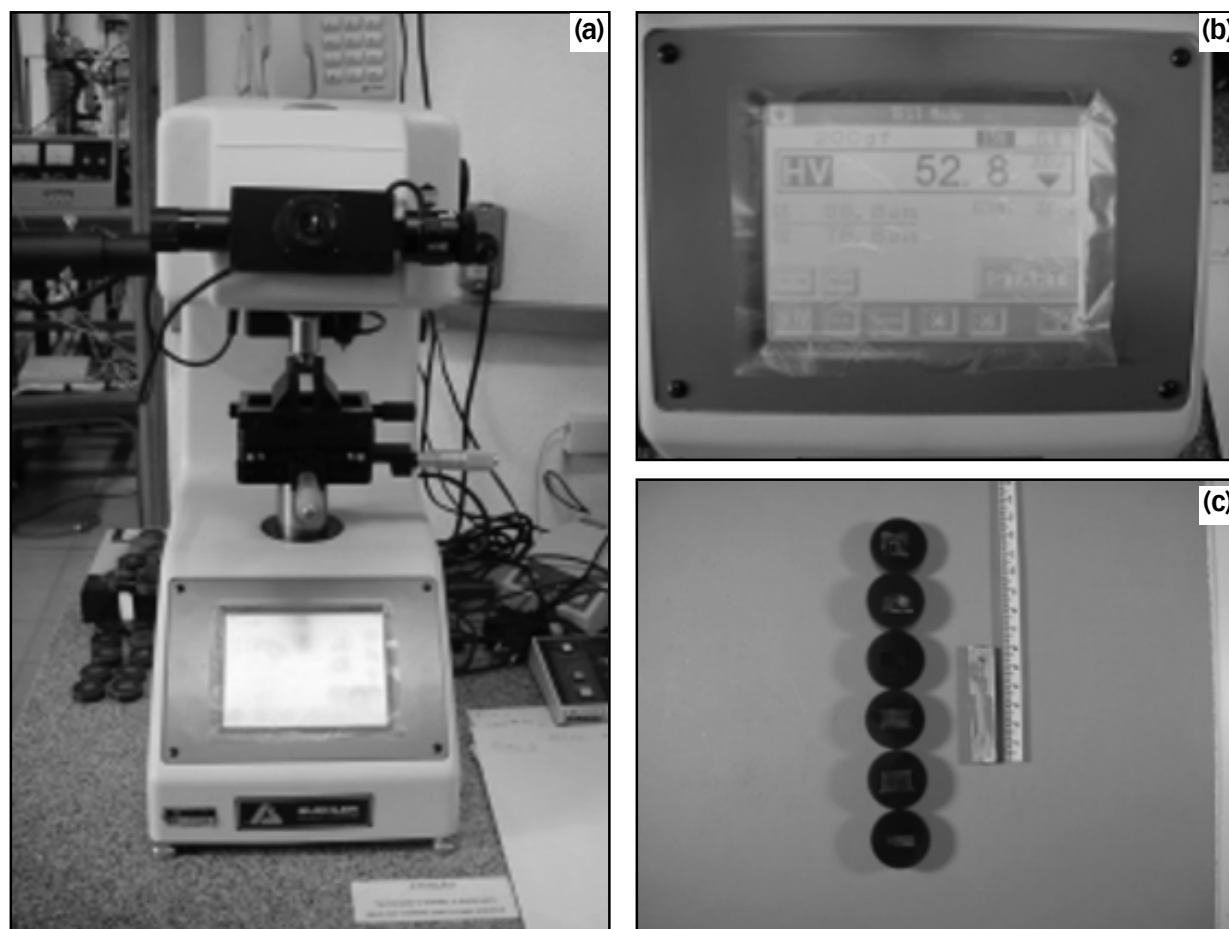
FIGURA 1: (a), (b): Microdurómetro Buehler utilizado para realizar las mediciones de microdureza, (c): Secciones de una probeta donde se realizaron las mediciones de microdureza.
