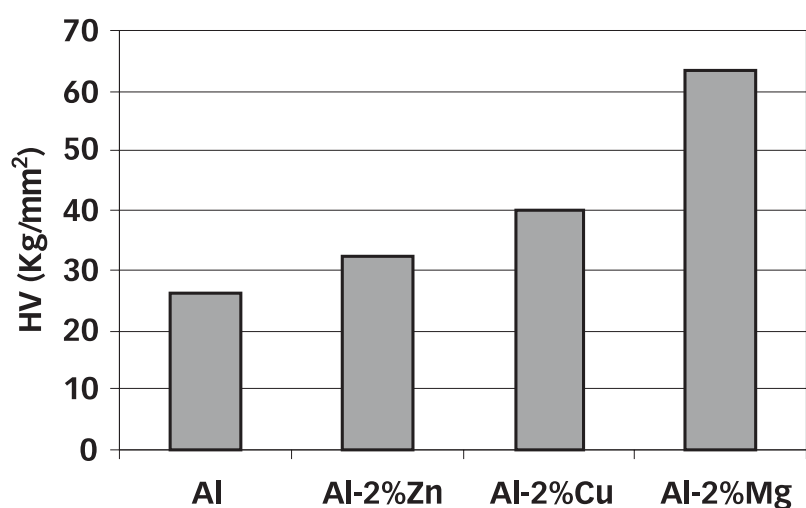
FIGURA 5: Valores de microdureza para una misma concentración de elemento aleante utilizando una carga de 100 g.
